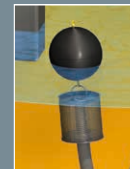
3 Stufe 3 schwimmender Ansaugfilter zur Wasserentnahme auf optimalem Niveau
