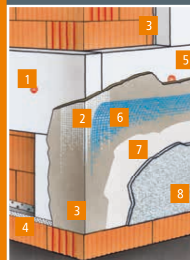
5 EPS-Dämmplatte
